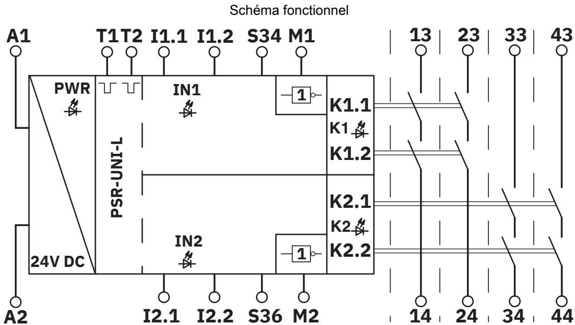
Schéma fonctionnel
