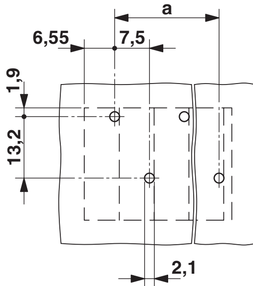
Bohrplan/Lötpadgeometrie
