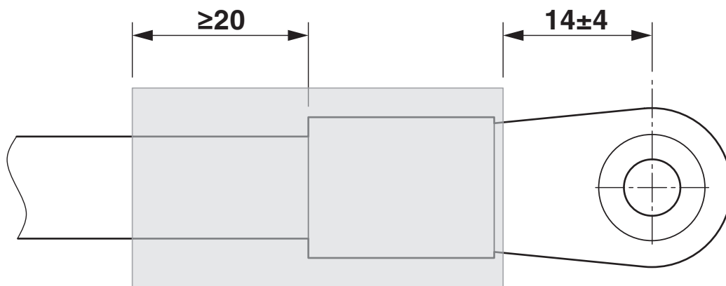
Maßzeichnung
