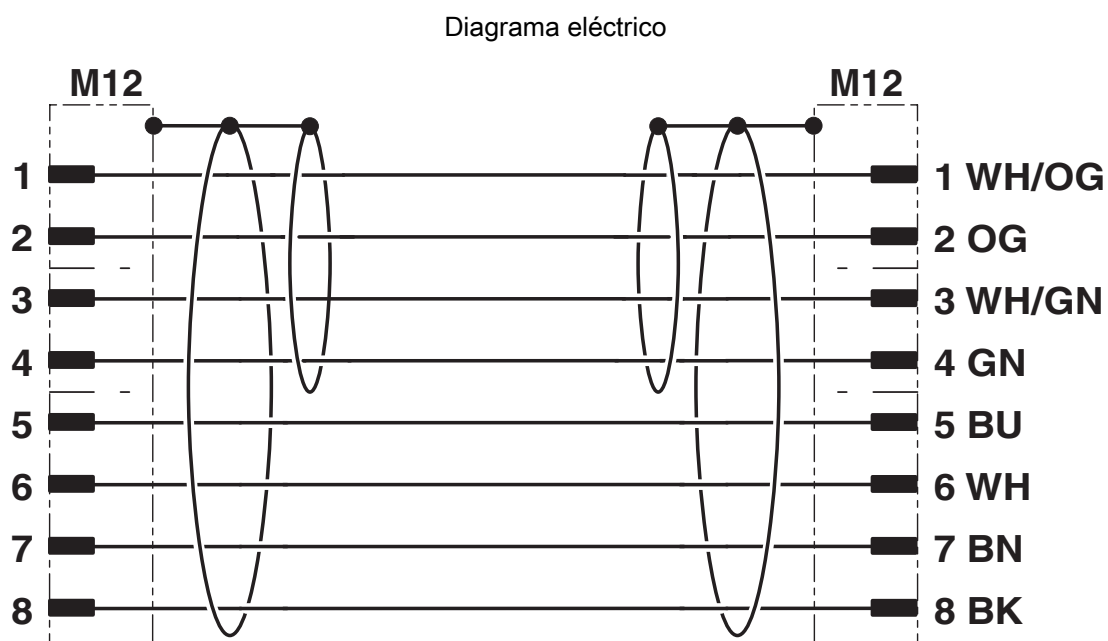
Ocupación de contactos de los machos M12
