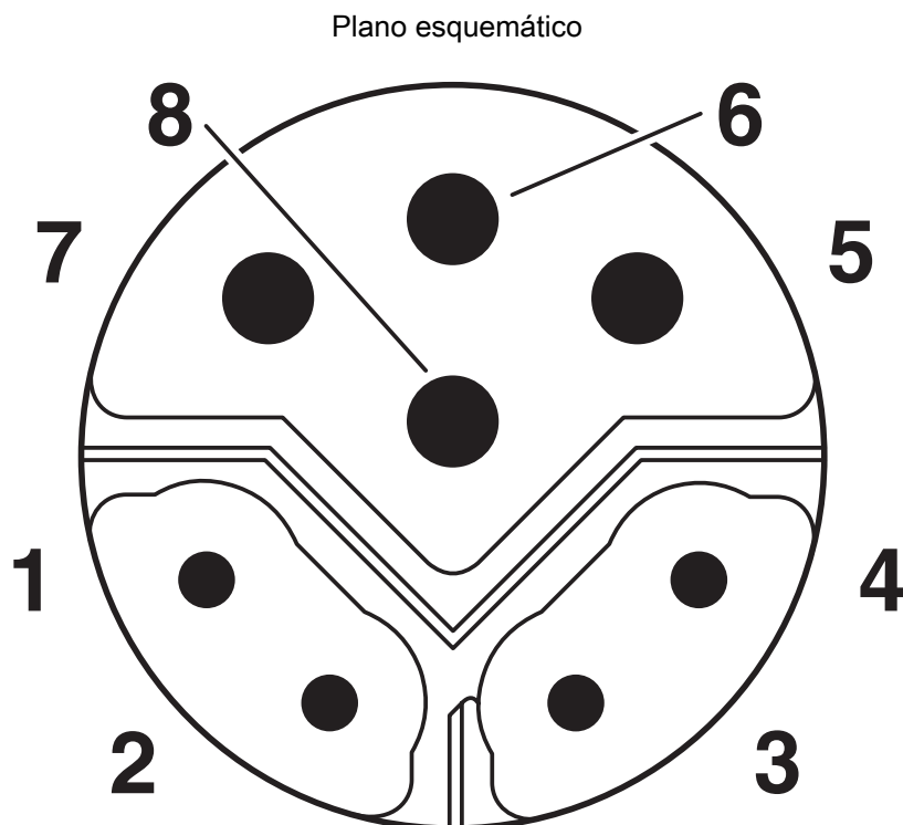
Esquema de polos conector híbrido M12 de 8 polos, codificado Y, vista lado macho
