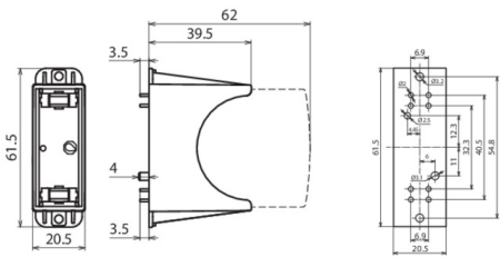
Dimensiones del DG PCB 385
