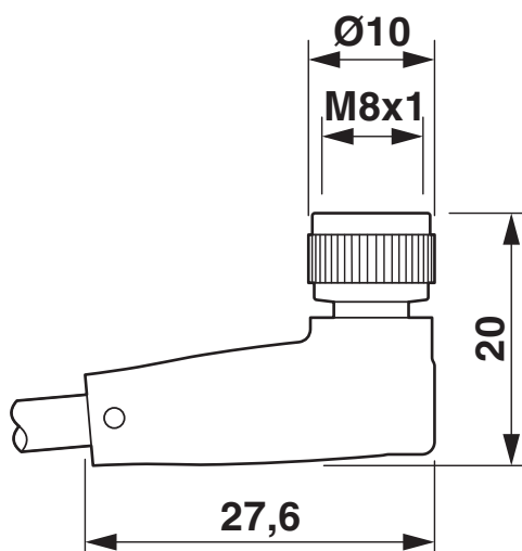
Dessin coté
