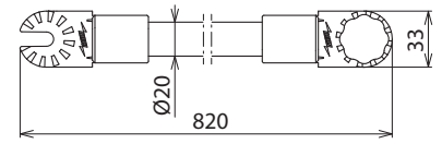
Maßbild ISV 820 ZK 123 SN7742
