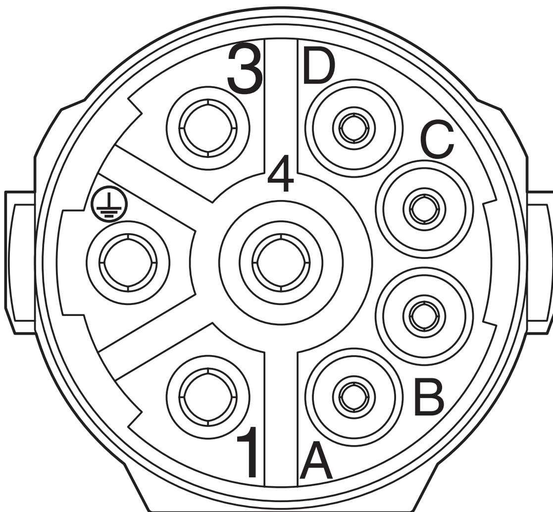
Schemazeichnung
