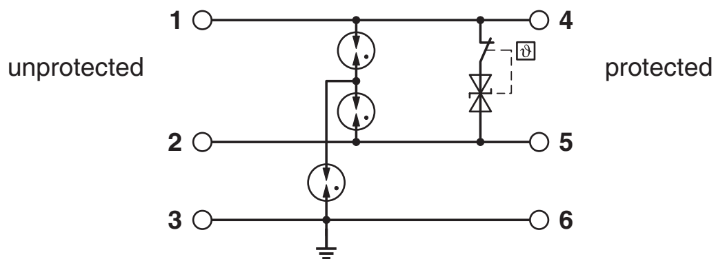
Diagrama eléctrico
