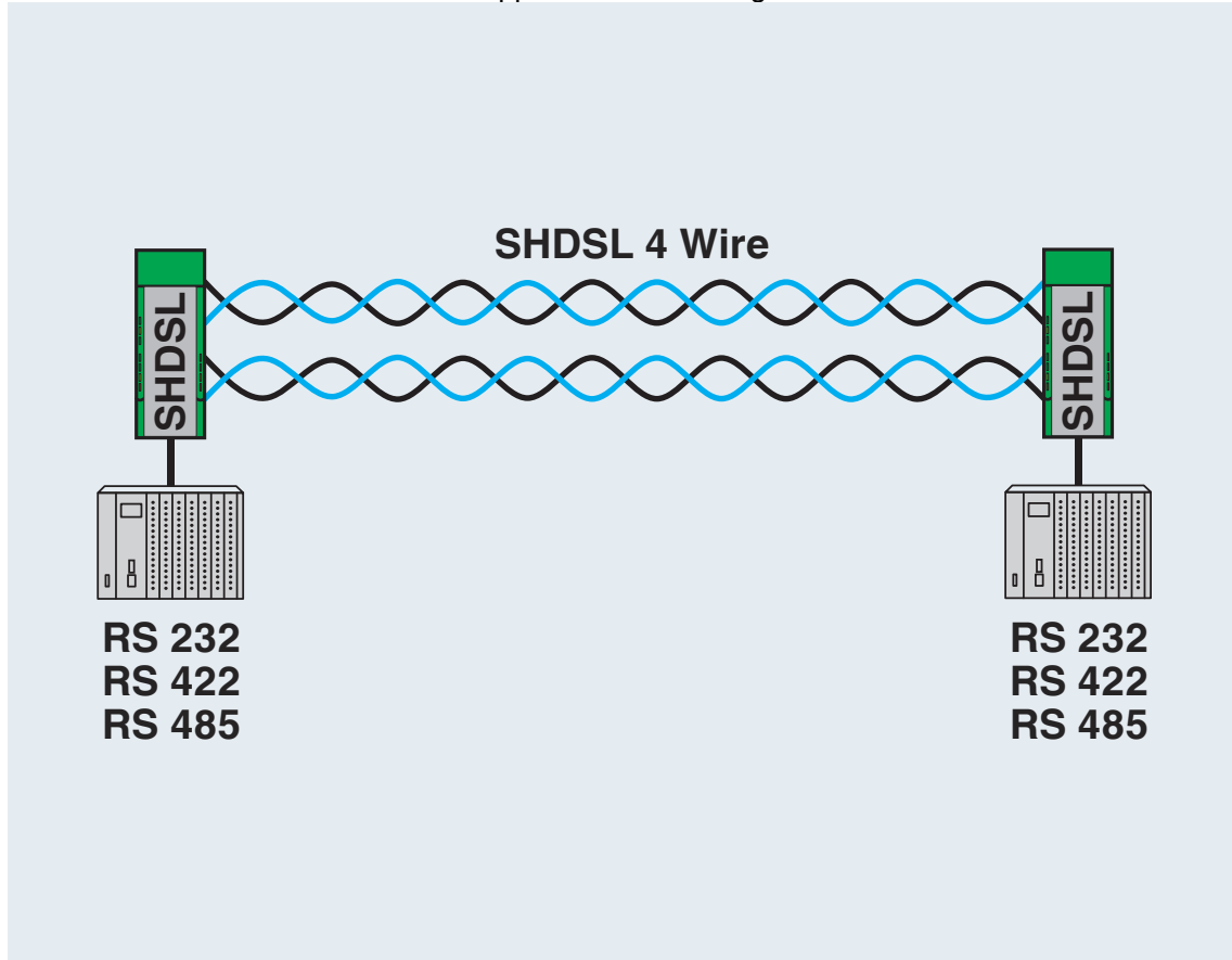
Punkt-zu-Punkt-Verbindung (4-Draht)
