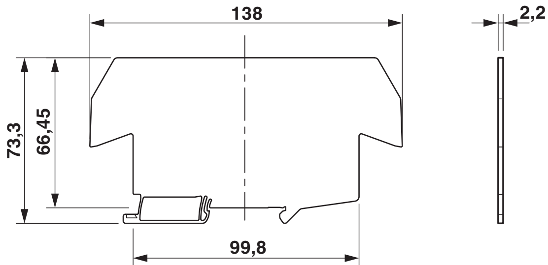
Dessin coté
