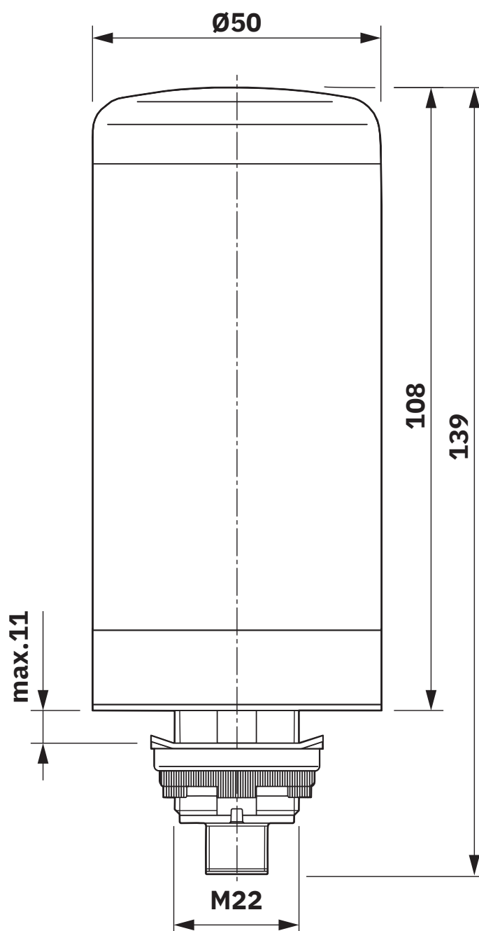
Dessin coté
