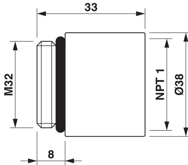
Maßzeichnung
