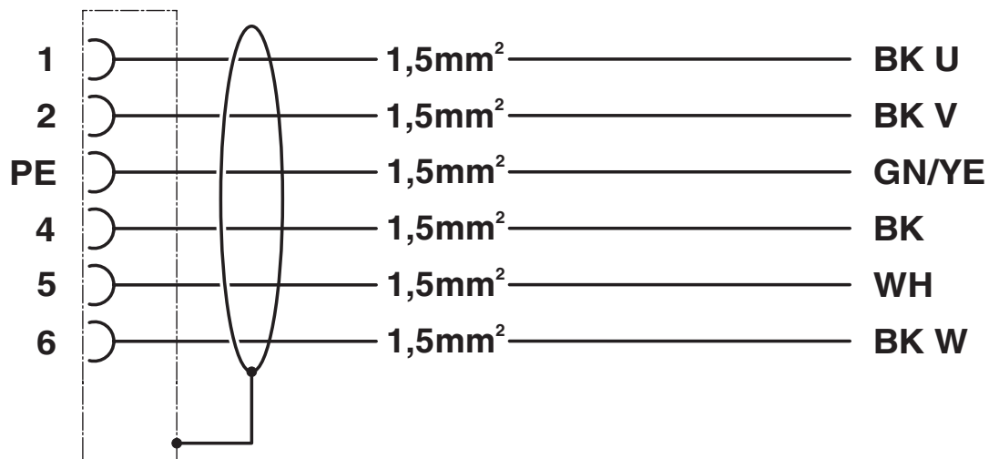
Schaltplan
