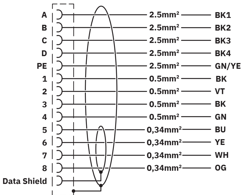
Diagrama eléctrico
