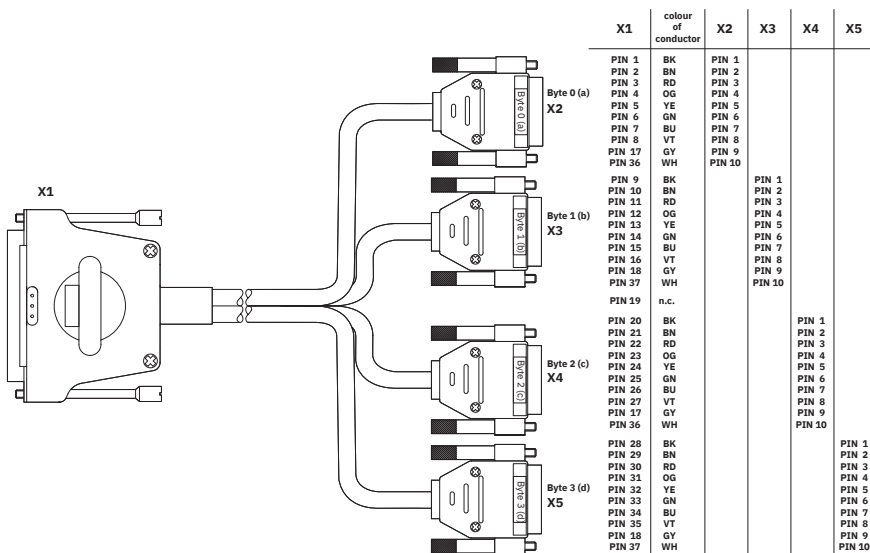
Schaltplan
