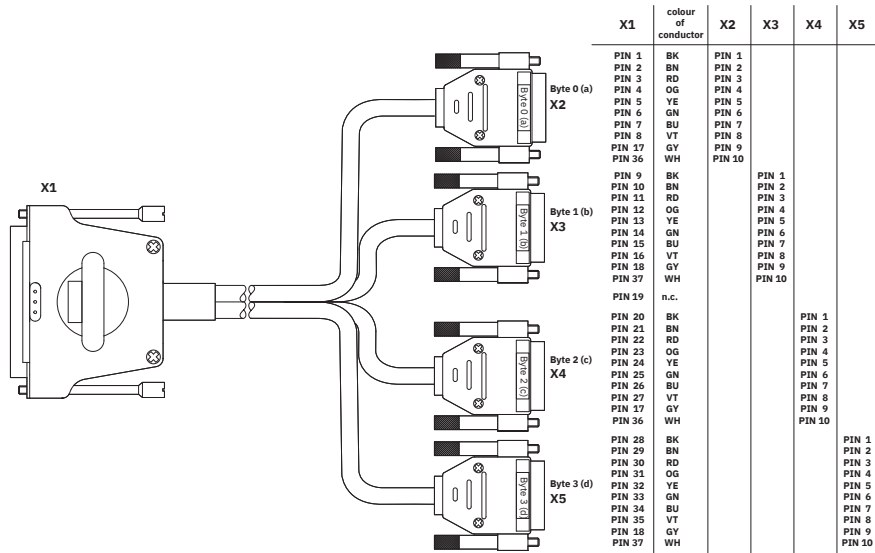
Diagrama eléctrico
