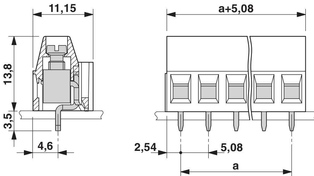
Maßzeichnung
