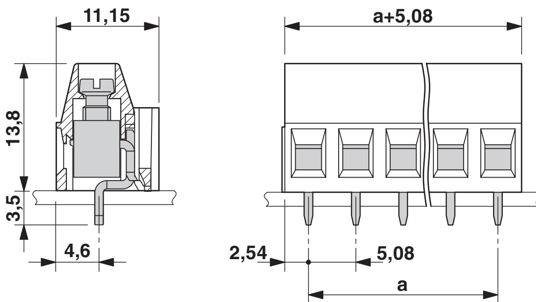
Dessin coté
