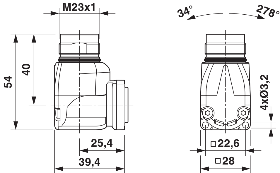
Maßzeichnung
