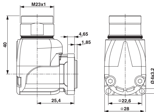
Maßzeichnung
