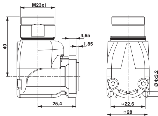
Dessin coté
