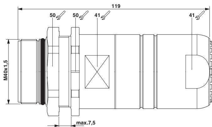
Maßzeichnung
