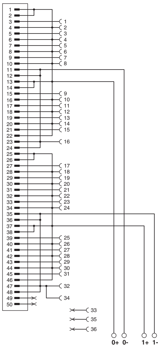
Schéma de connexion
