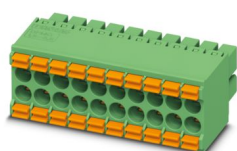
La figura muestra una variante de 10 polos con 20 contactos
