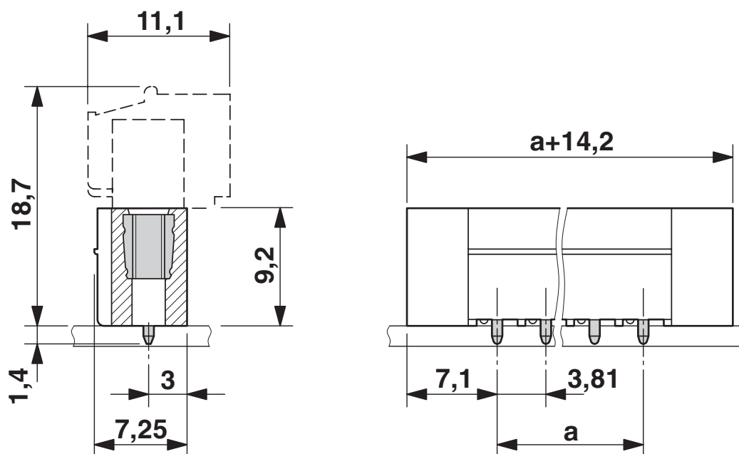
Dessin coté
