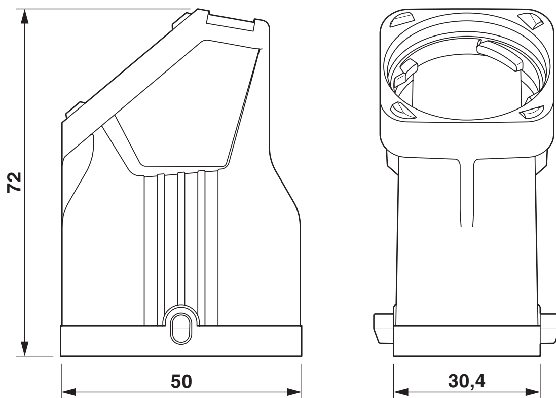
Dessin coté
