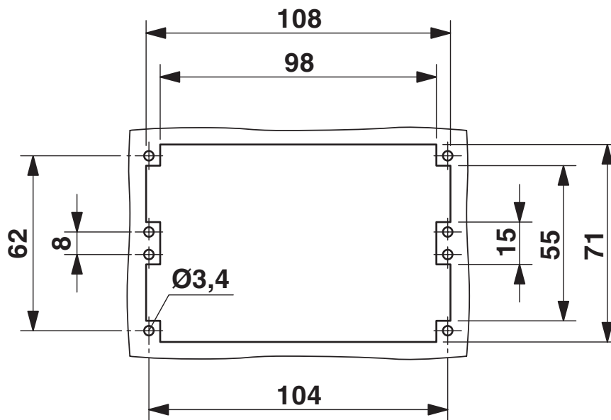
Dessin coté
