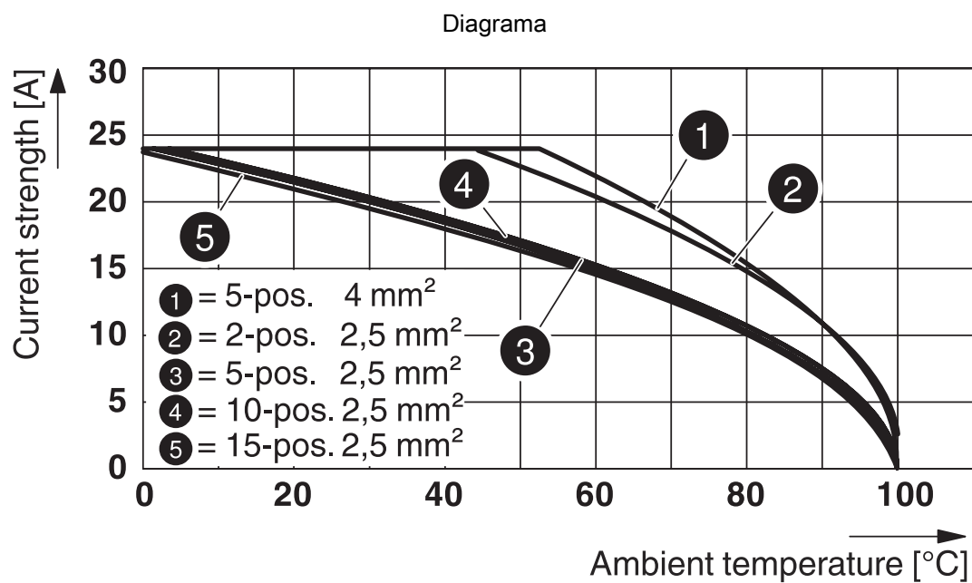
Diagrama eléctrico
