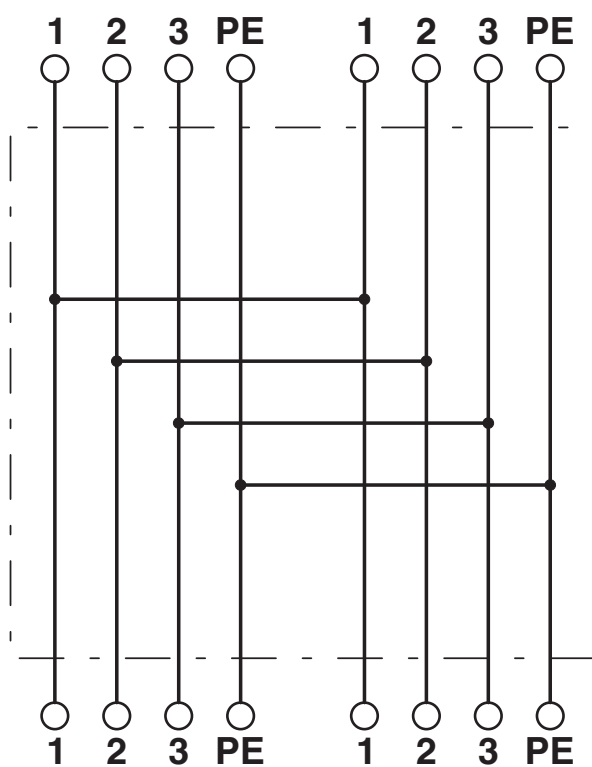
Diagrama eléctrico
