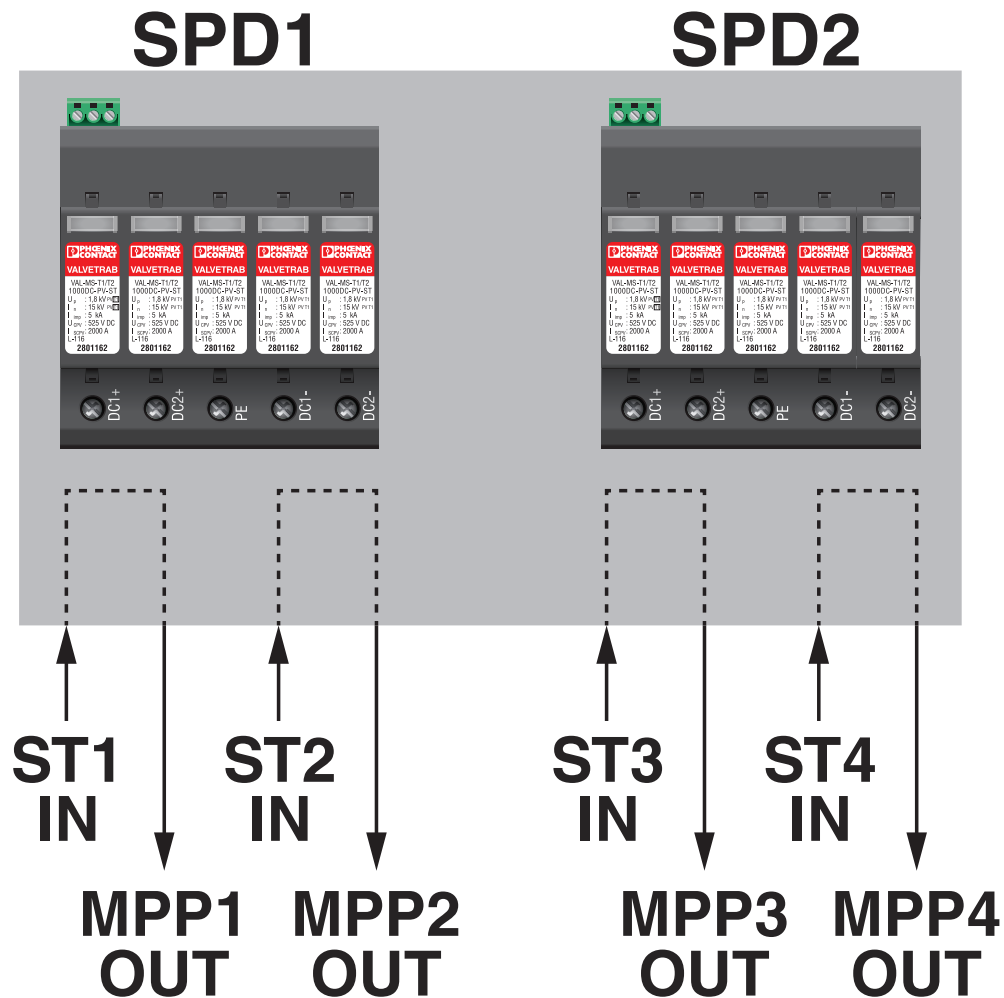
Anschlusszeichnung
