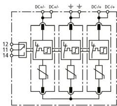
Esquema del DCU 2 YPV 1100 3M 1S MC4 FM
