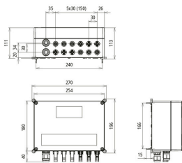
Dimensiones del DCU 2 YPV 1100 3M 1S MC4 FM
