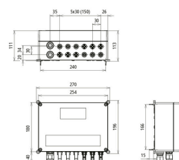
Dimensioni DCU 2 YPV 1100 3M 1S MC4 FM
