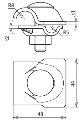
Maßbild MVK 8.10 16 FRM10X40 STTZN
