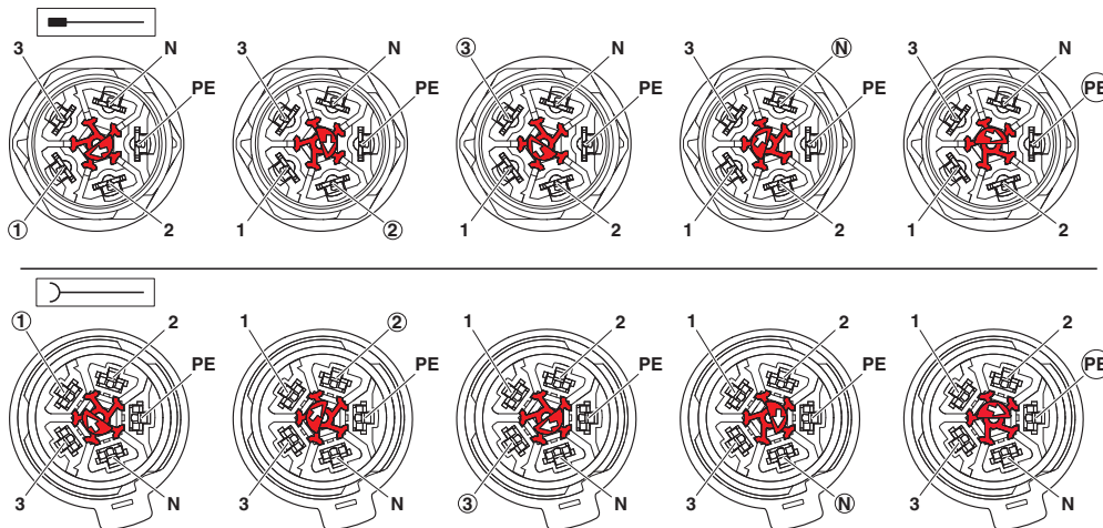
Funktionszeichnung
