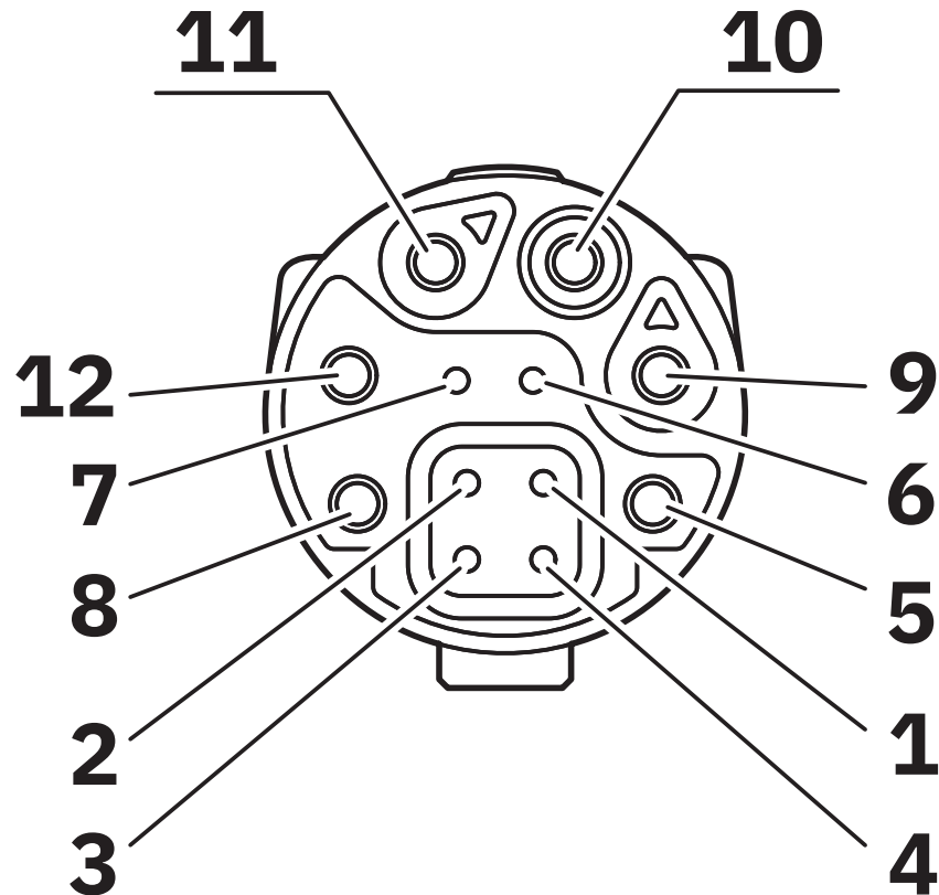
Schemazeichnung
