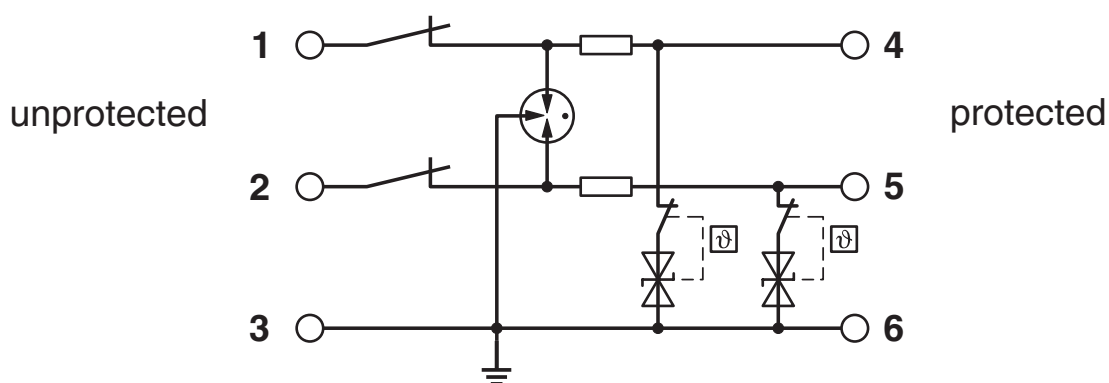
Diagrama eléctrico
