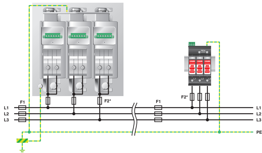
Applikationszeichnung
