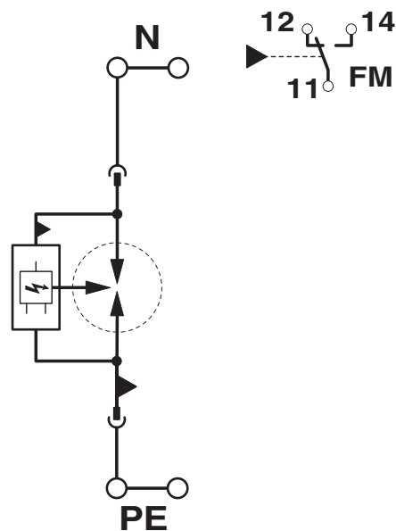
Schaltplan
