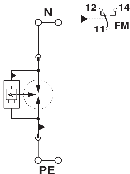
Diagrama eléctrico
