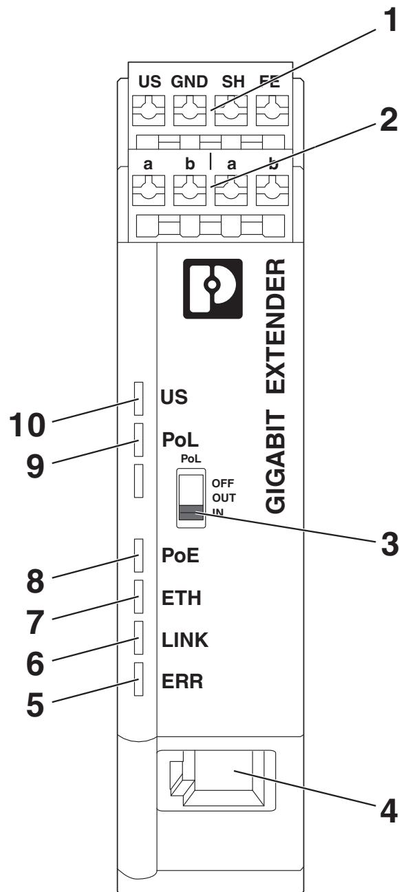
Schemazeichnung
