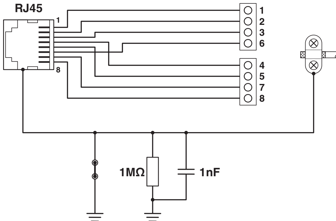
Diagrama eléctrico
