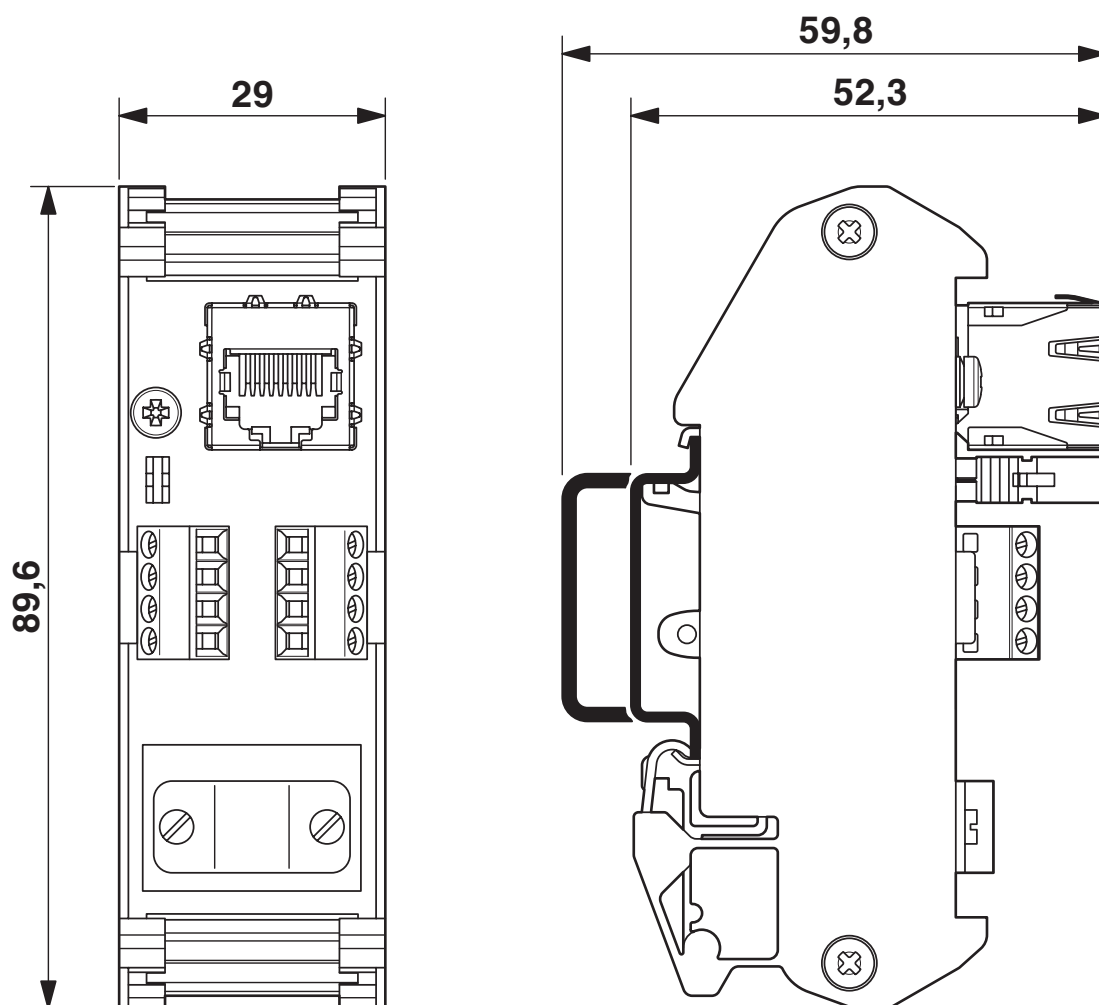
Dessin coté
