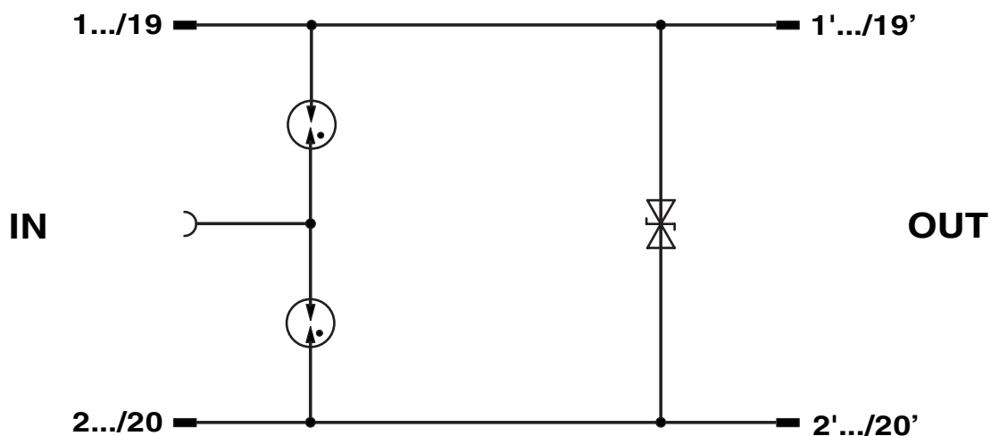
Diagrama eléctrico
