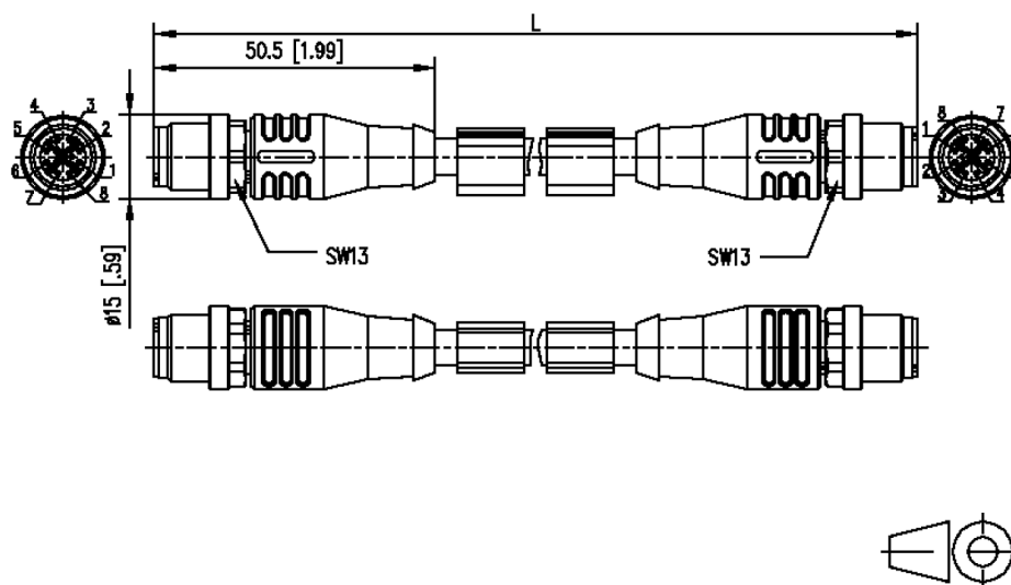
M12 plug
