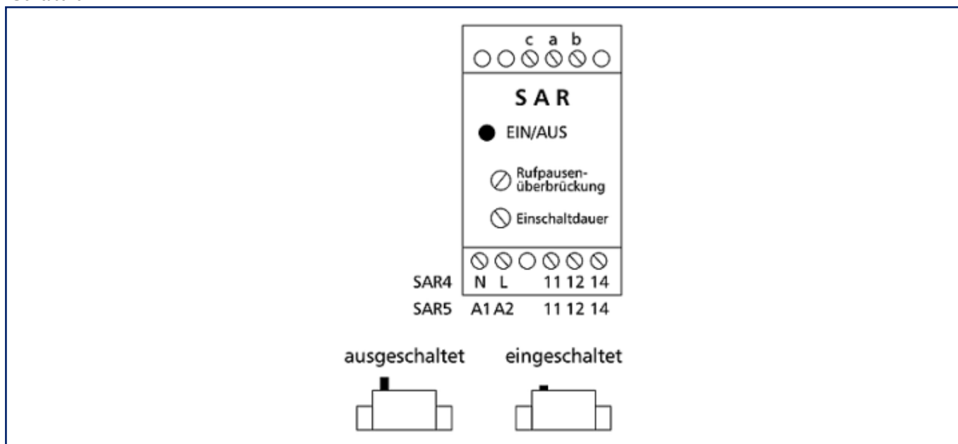
Schaltbild
