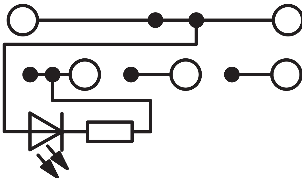
Diagrama eléctrico
