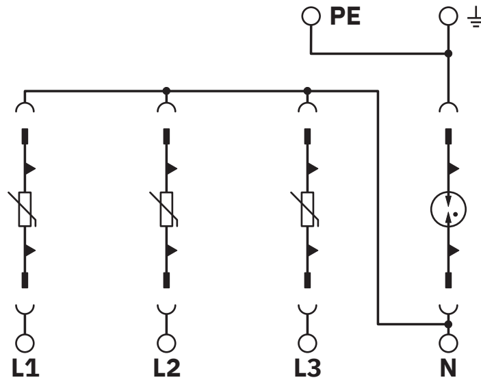
Diagrama eléctrico
