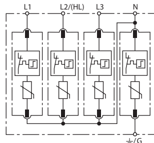
Prinzipialschaltbild DG MU 3PH 480 4W+G
