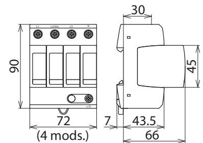
Maßbild DG MU 3PH 480 4W+G
