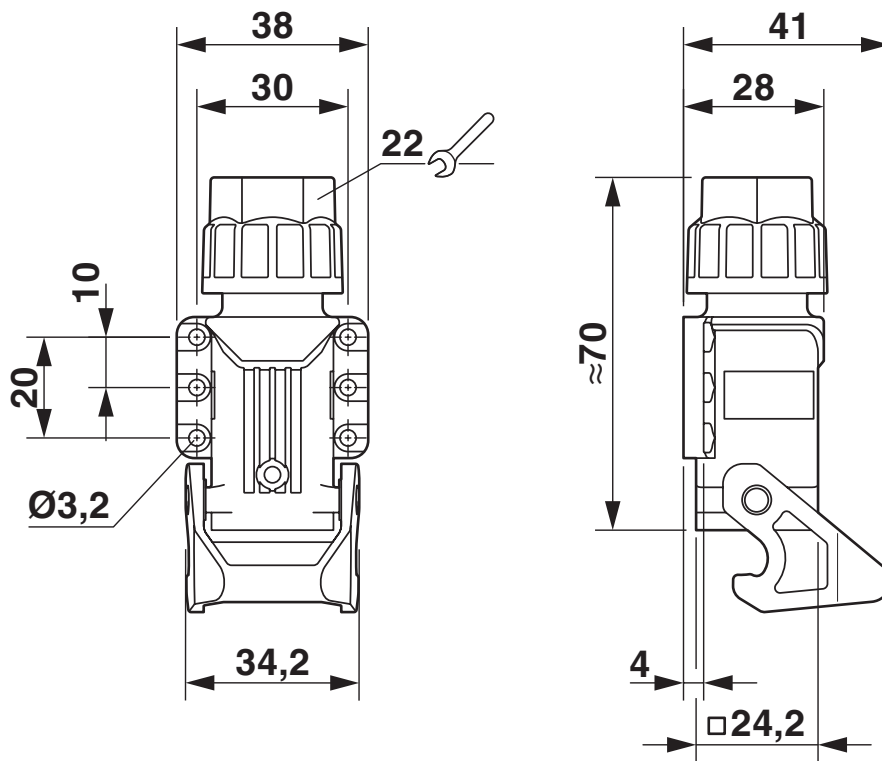
Maßzeichnung
